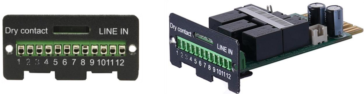
Внешний вид мини карты релейного интерфейса
