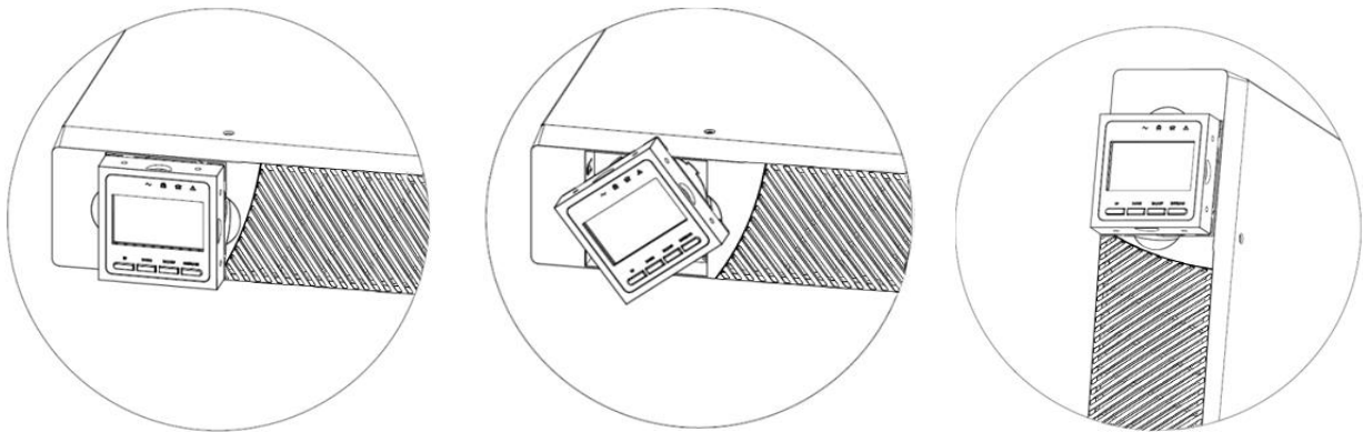
Рисунок 12 Поворот ЖК-дисплея ИБП при напольной установке
